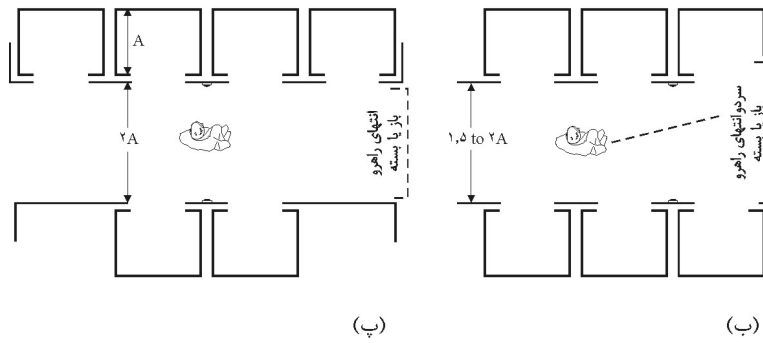
جانمایی شش آسانسور (ب)
