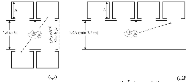
جانمایی چهار آسانسور (الف)
