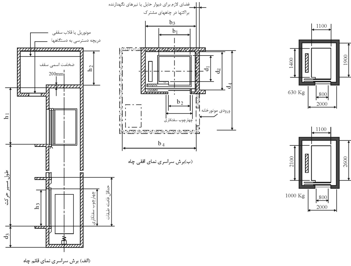
شکل ۱-۳ طرح اولیه معماری آسانسورهای الکتریکی ساختمان‌های مسکونی. (دسته دوم)
