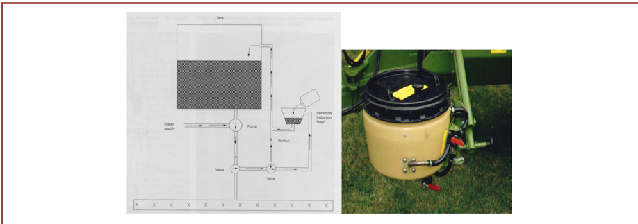
شکل ۱۰- پیمانه القائی جهت پرکردن سم پاش
