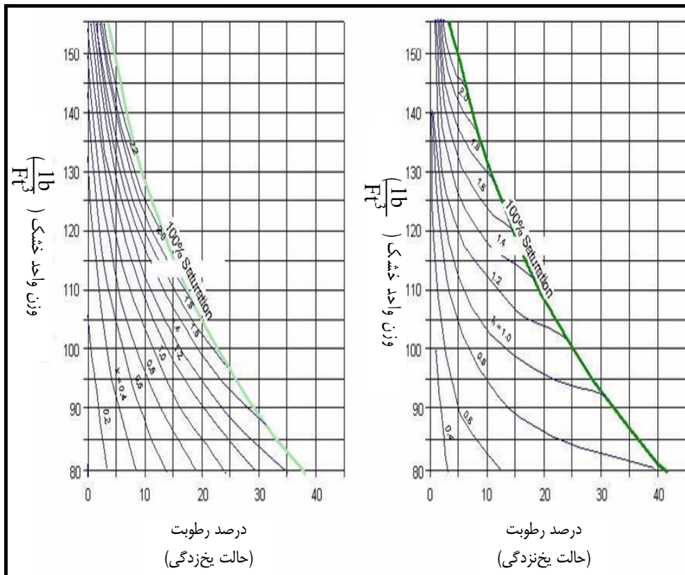
شکل پ. ۱-۵- متوسط ظرفیت انتقال حرارتی برای خاک‌های گرانولی در دو حالت یخ‌زدگی و یخ‌زدگی (برگرفته از Kersten, 1949 and Air Force, 1966)
