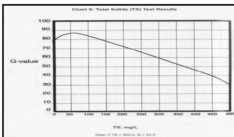
شکل پ.۵-۷- نمودار تعیین کیفیت آب بر اساس کل مواد جامد
