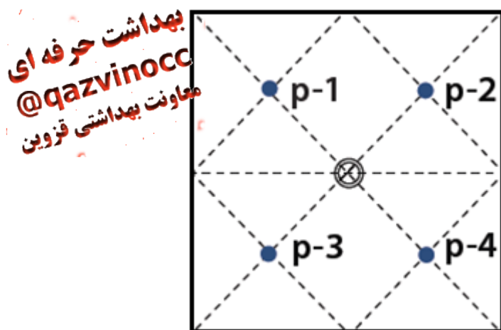
شکل (۱۵) الگوی یکم در اندازه‌گیری روشنایی عمومی داخلی
