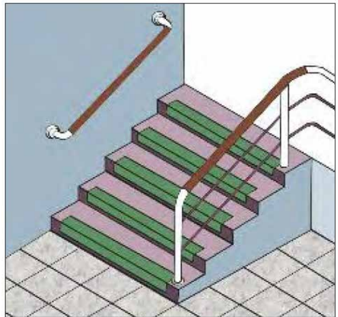
شکل ۳-۲: برای پیشگیری از سرخوردگی روی سراشیبه ها و پله ها اقداماتی انجام دهید. مواد دارای اصطکاک بالا که در لبه پله ها گذاشته شده می تواند کمک کند.
