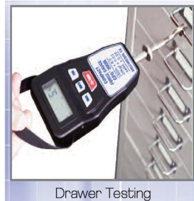
شکل ۲۲: دینامومتر دستی (نیروسنج هل دادن/کشیدن).
