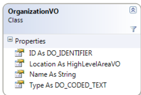
شکل ۷ - کلاس OrganizationVO
