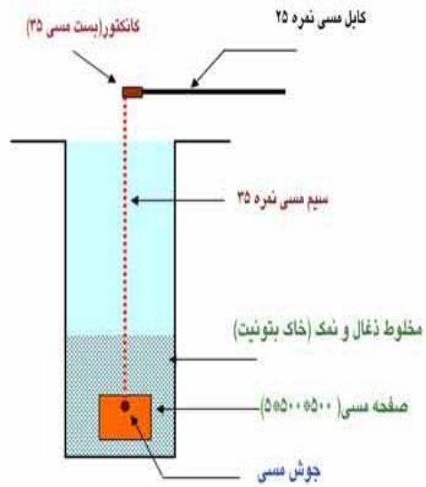
نمای کلی سیستم اتصال زمین
